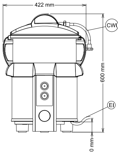
Вид спереди
